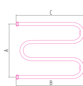
М-образный 500x650 **0007-5065
