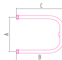
П-образный 320x500 00-0003-3245
